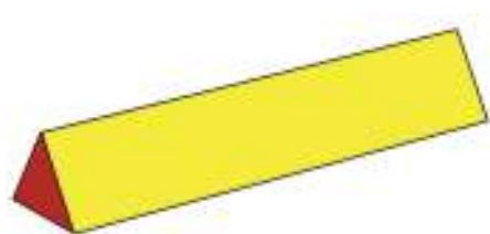
Prisma Segitiga
