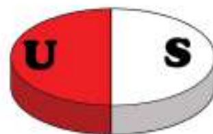
Magnet Lingkaran
